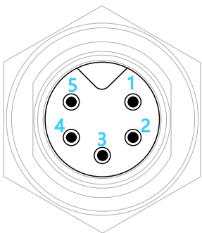
图 3 触发接口图
