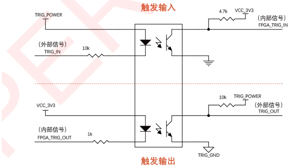
图 4 触发电路参考图
