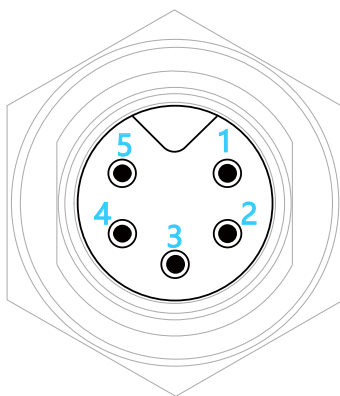
图 2 触发接口图
