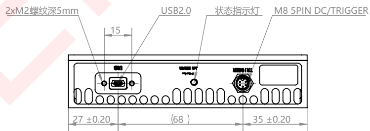
图 4 FM830-RI 尺寸图 (单位: mm)
