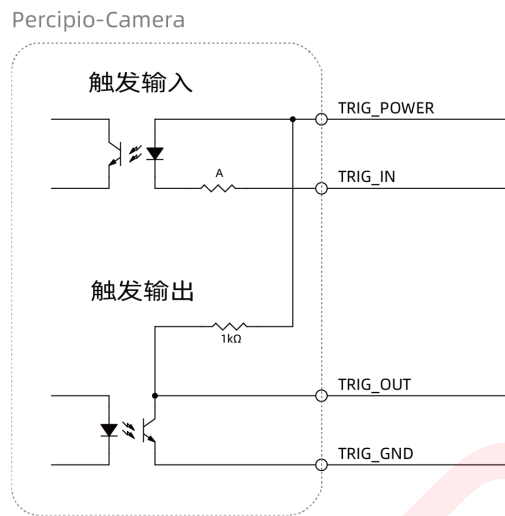
图 3 触发电路原理图（下降沿）
